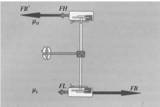
图 15.31 在不同路面上加速时作用在汽车车轮上的力
