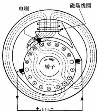
图 1.4 三刷发动机
