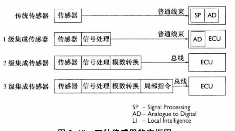
图 2.68 四种传感器的方框图
