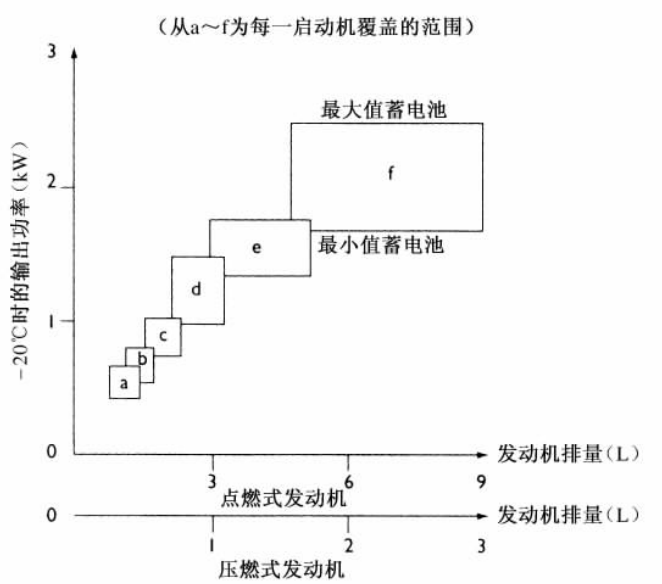
图 7.5 启动机所需的功率与发动机型号之间的关系
