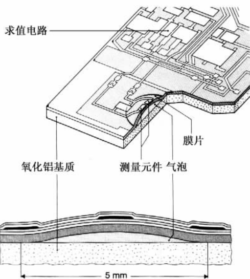
图 2.65 厚膜压力传感器
