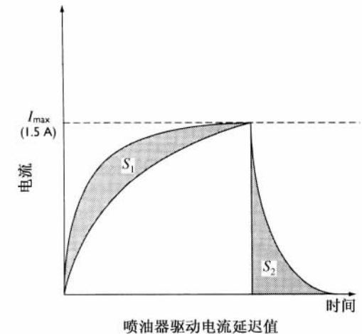
图 10.51 喷油器驱动电流曲线
