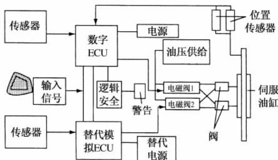
图 15.15 主动转向系统的基本组成
