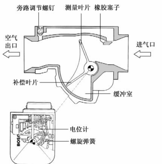
图 2.54 空气流量计(叶片型)
