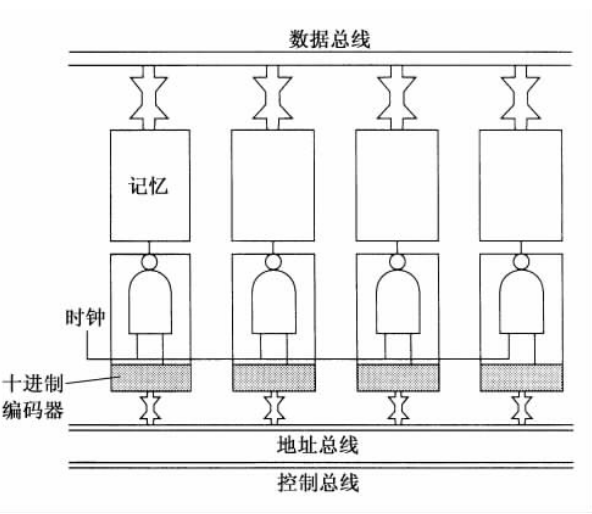
图 2.37 具有地址总线和译码器的 4 位存储器
