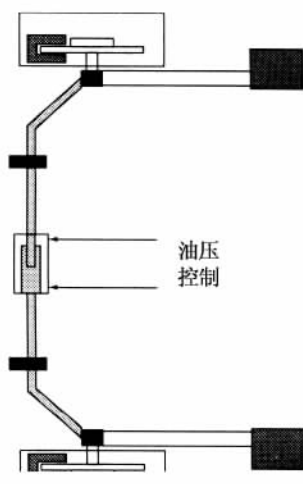
图 15.17 主动降低侧倾的位置控制
