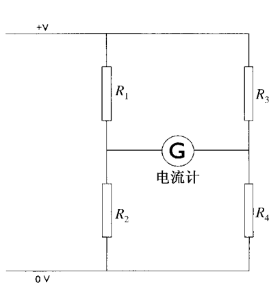
图 2.20 惠斯顿电桥
