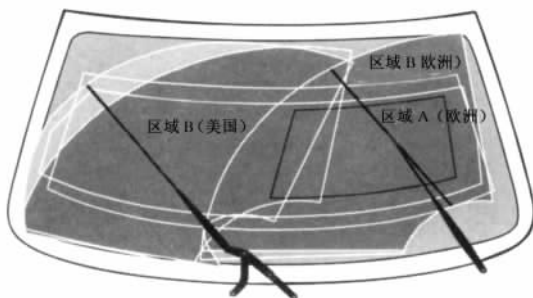
图 12.2 刮水区
