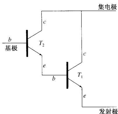
图 2.25 达林斯顿管
