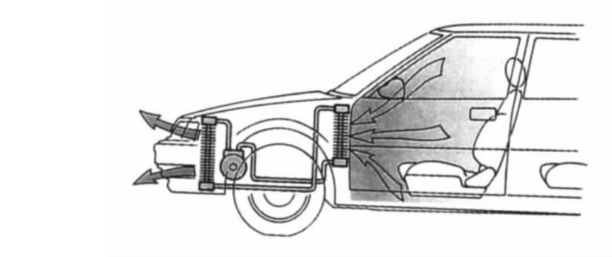
图 14.9 空调系统的工作过程
