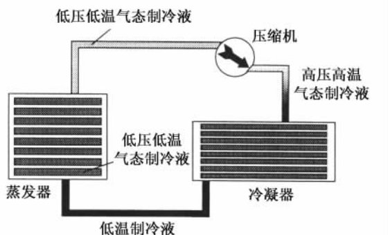
图 14.7 空调系统制冷循环图
