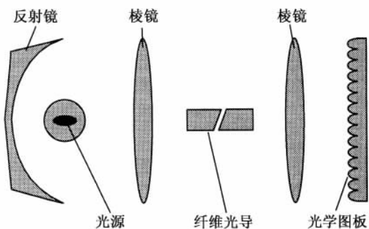
图 11.27 气体放电灯光通过特制棱镜进入并离开光导的结构示意图
