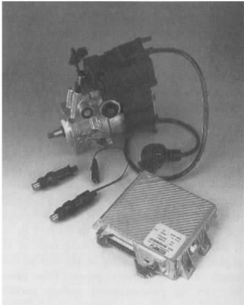
图 9.38 电控分配式喷油泵
