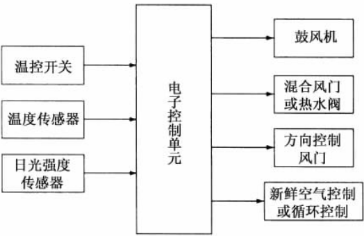
图 14.6 电子控制加热系统框图
