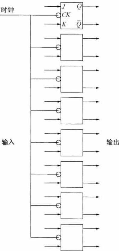
图 2.36 触发器构成的 8 位寄存器
