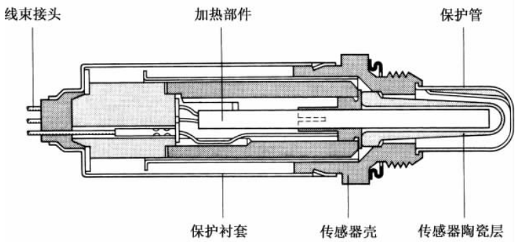
图 2.63 氧传感器
