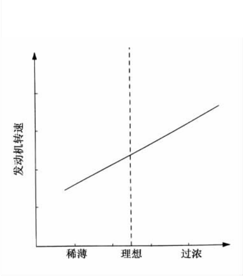
9.15 在简易阻风门式化油器中,吸入空气流中的燃油量并不与空气量的增长成线性变化
