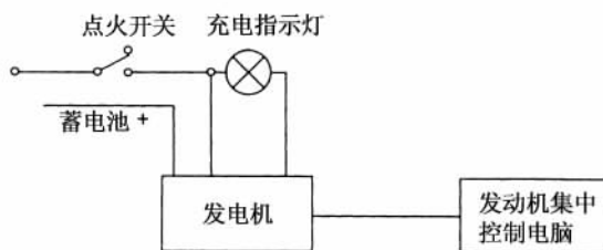
图 6.31 发电机与发动机集中控制电脑之间的连接关系图
