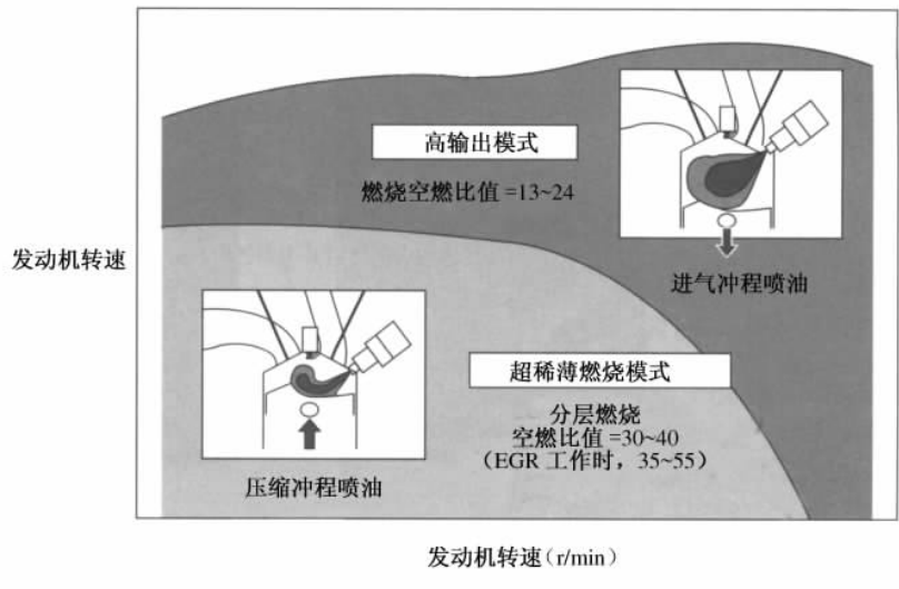
图 10.24 GDI 发动机的两种燃烧模式
