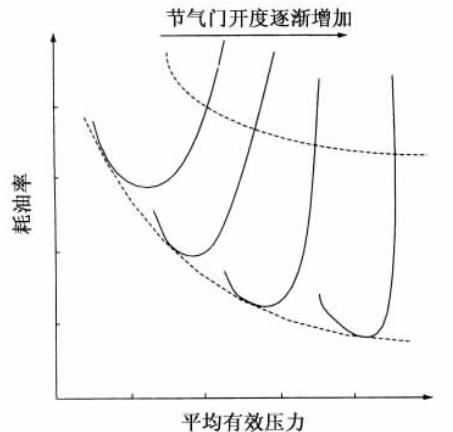
图 9.8 不同节气门开度下,混合气浓度特性曲线
