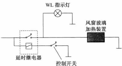
图 14.11 风窗玻璃加热装置
