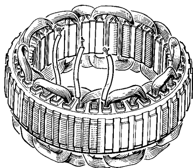
图 6.6 定子结构示意图
