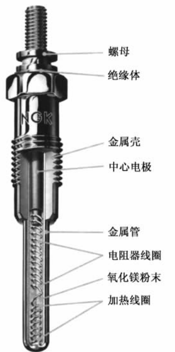
图 9.41 典型的柴机电热塞
