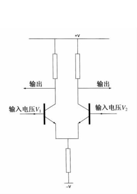
图 2.17 直流放大器(加长尾)
