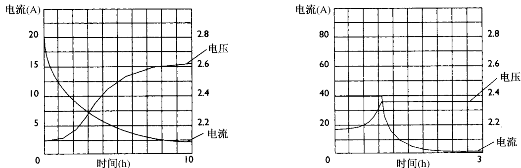
图 5.4 蓄电池的两种充电方式显示充电电压与充电电流
