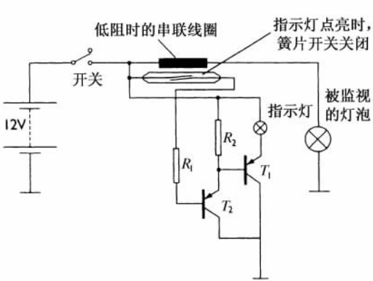
图 13.12 灯泡烧毁警告电路
