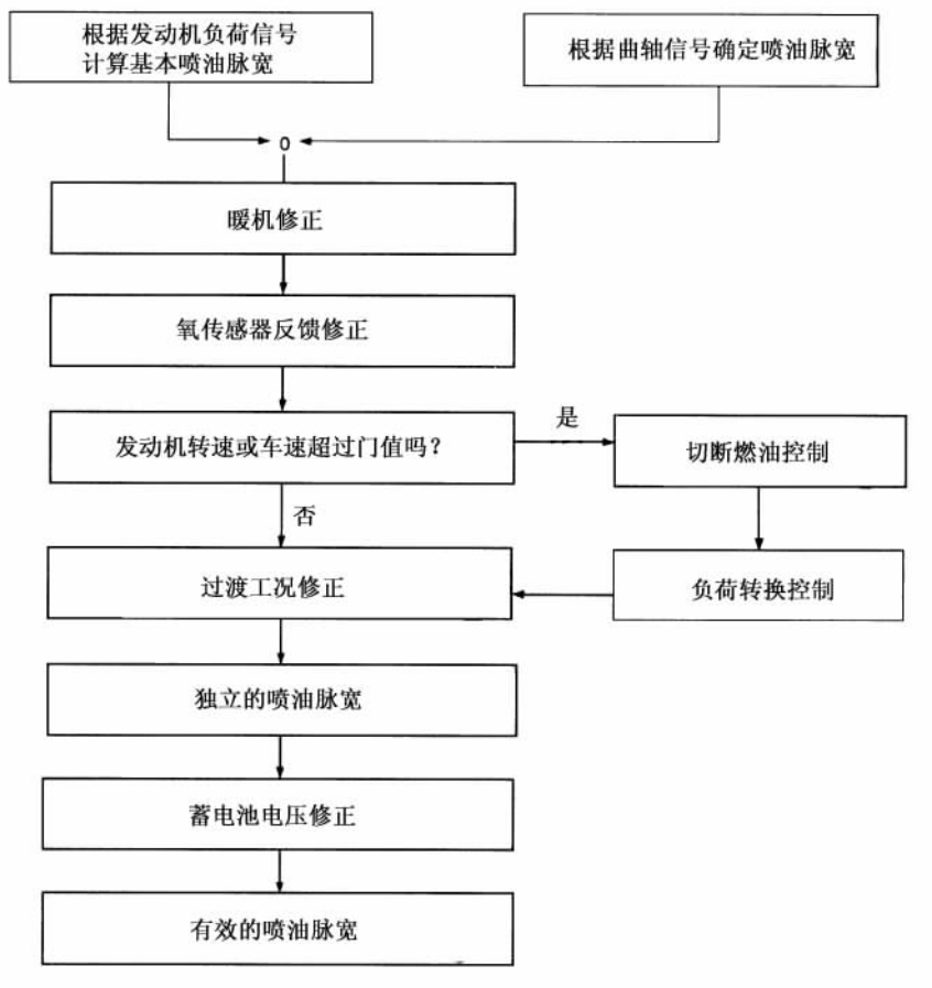
图 10.55a 喷油脉宽计算流程框图
