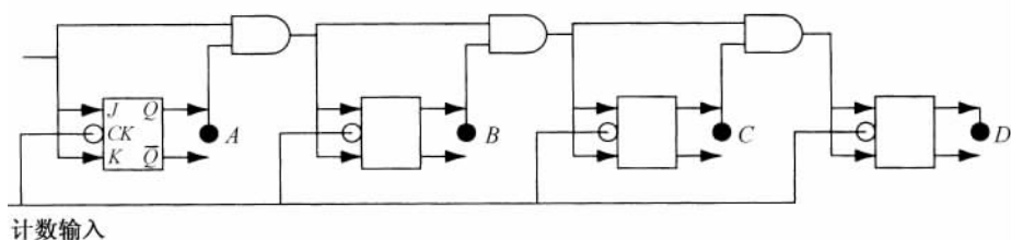
图 2.35 4 位同步计数器
