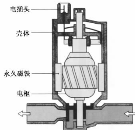
图 9.28 旋转式怠速执行器
