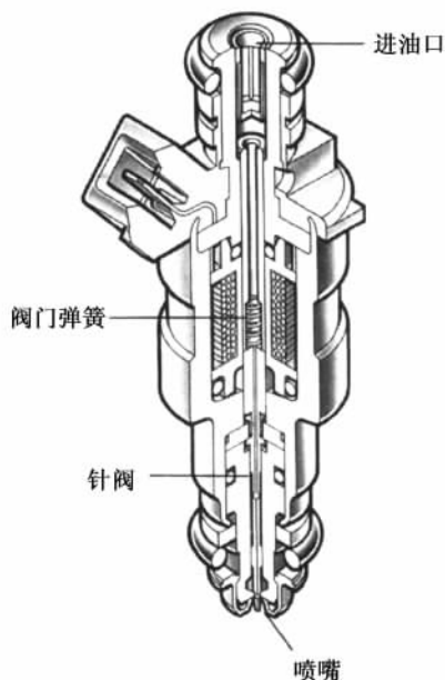
图 9.48 喷油器
