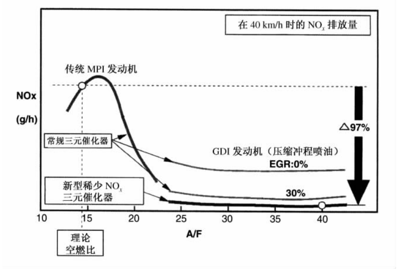
图 10.33 不同空燃比下 NO x 的排放量
