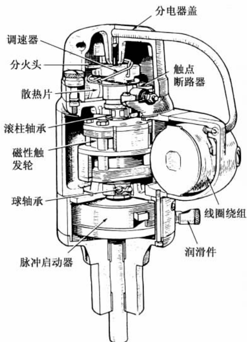
图 1.7 卢卡斯 6VRA 永磁发电机的局部示意图
