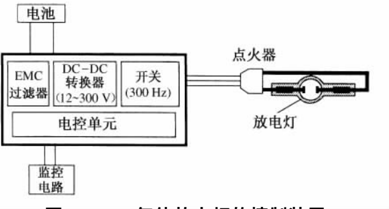
图 11.16 气体放电灯的控制装置
