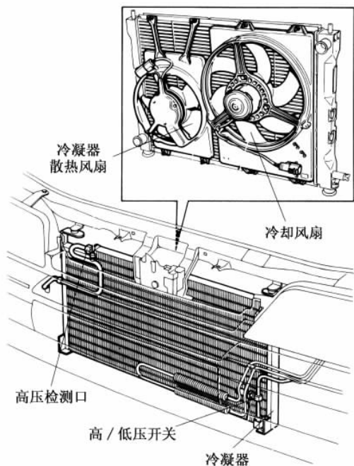
图 14.14 冷凝器
