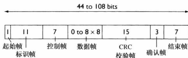
图 4.23 一个 CAN 命令是由起始帧、标识帧、控制帧、数据帧、用于错误侦测的循环冗余检验帧、CRC 检验帧、确认帧以及结束帧组成
