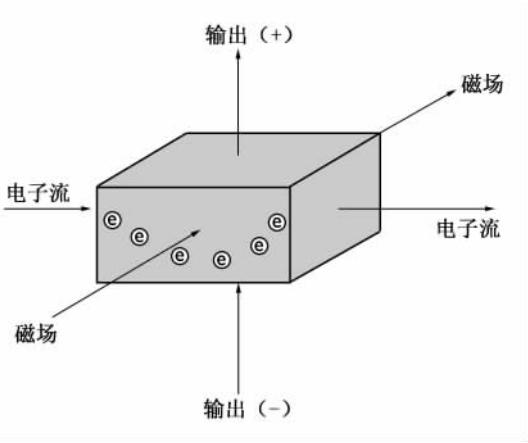
图 2.48 霍尔效应原理
