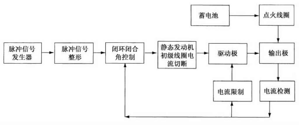
图 8.16 闭环闭合角控制系统
