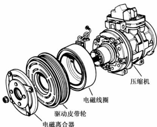
图 14.13 空调压缩机
