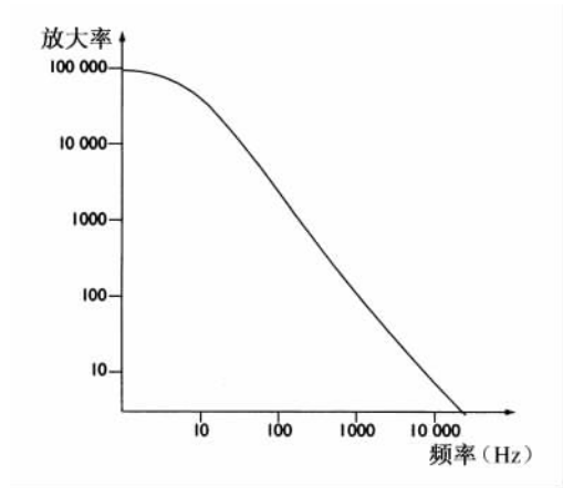
图 2.19 741 放大器的频率响应
