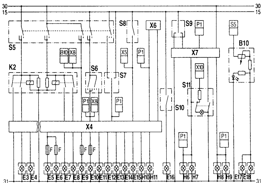
图 11.21 照明电路流程图
