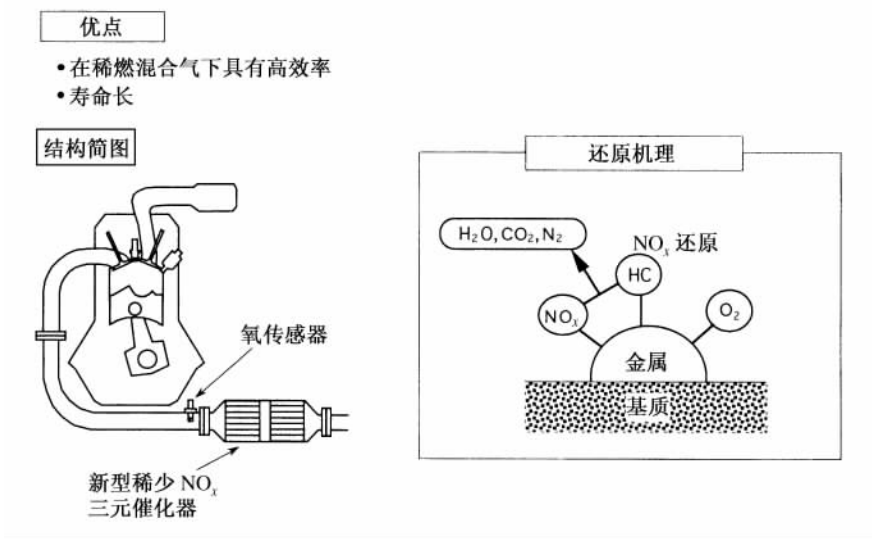
图 10.34 新型稀少 \text{NO}_x 三元催化器
