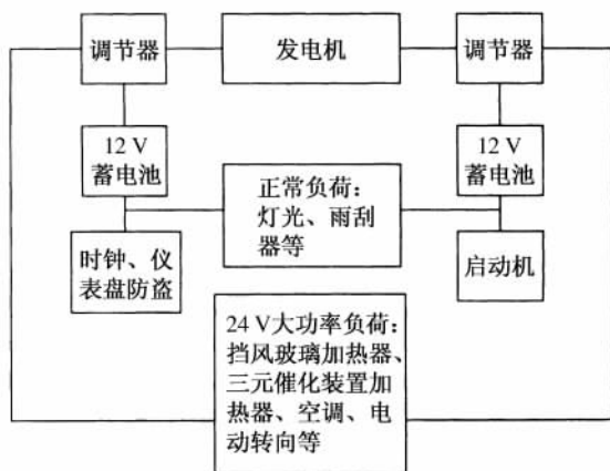
图 6.32 双路功率供给技术
