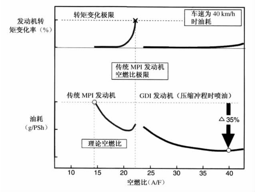
图 10.31 定速工况时 GDI 与 MPI 发动机的油耗和转矩对比
