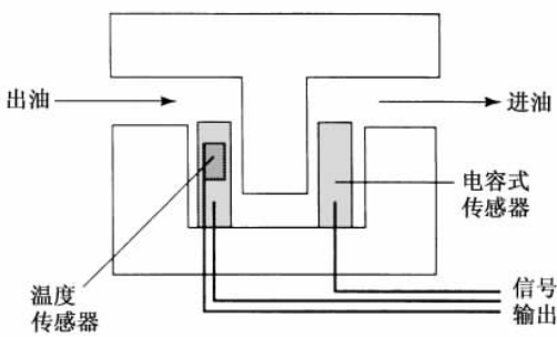
图 2.66 甲醇传感器
