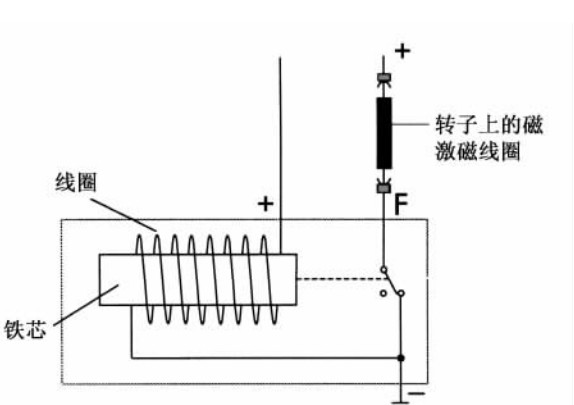
图 6.18 机械型电压调节器的工作原理
