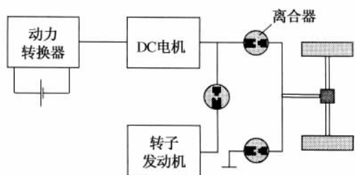
图 17.9 Nelco 并式混合动力驱动系统布置图
