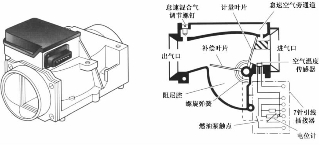
图 9.24 空气流量计
