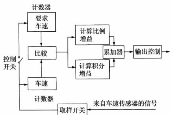
图 16.49 巡航控制系统的控制原理方框图
