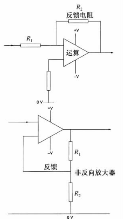
图 2.18 运算放大器反馈电路
