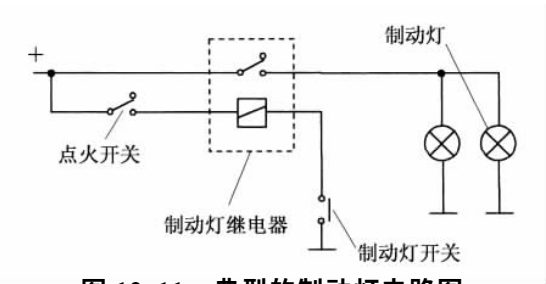
图 12.11 典型的制动灯电路图
