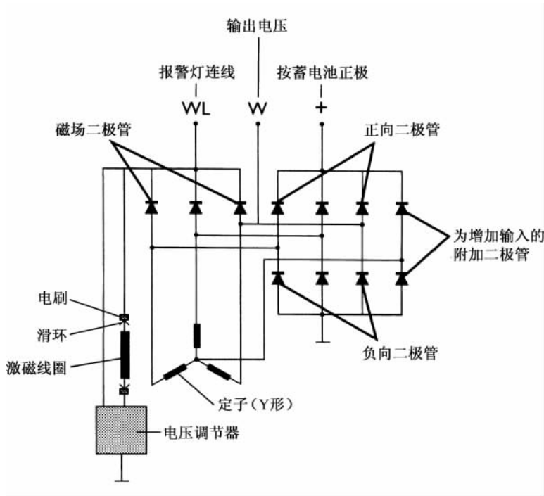
图 6.14 交流发电机的电路图
