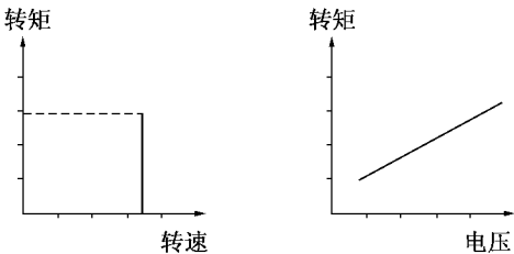
图 2.77 回动同步电机电路及速度转矩特性
