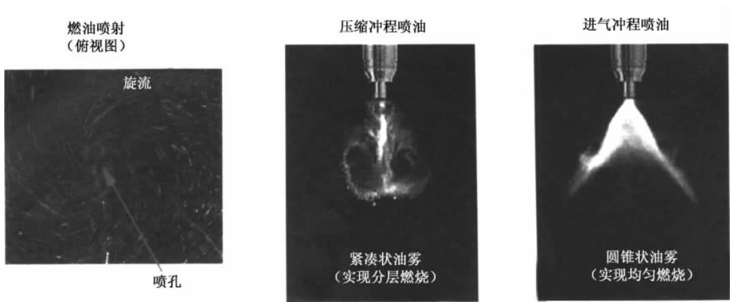
图 10.26 高压旋转式喷油器
