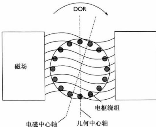
图 14.18 转子效应
