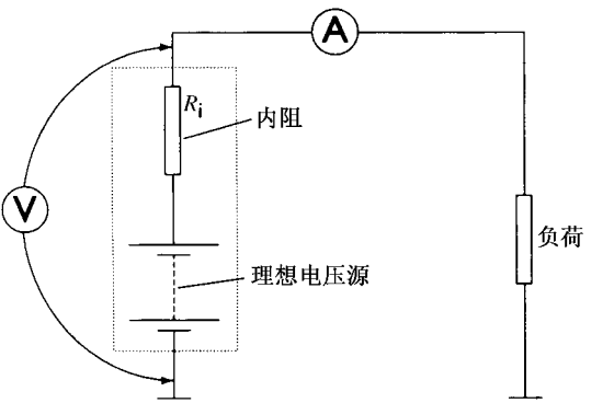
图 5.8 电源端电压随着负荷变化的等价电路
