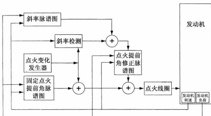
图 10.57 自适应点火控制方框图
