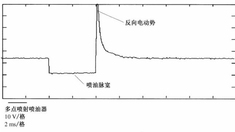
图 3.27 喷油器波形图
