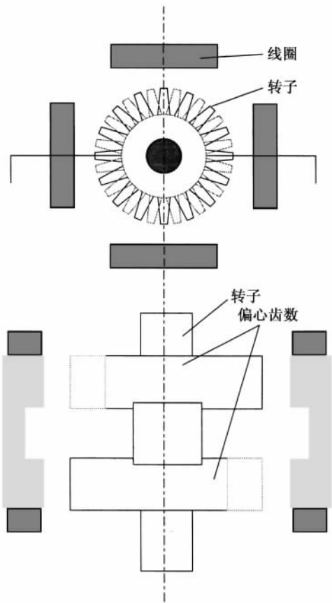
图 2.74 由极距移动的双定子步进电机
