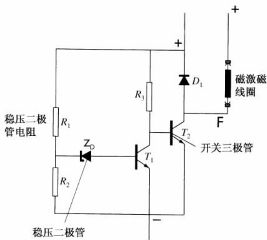
图 6.19 电子电压调节器
