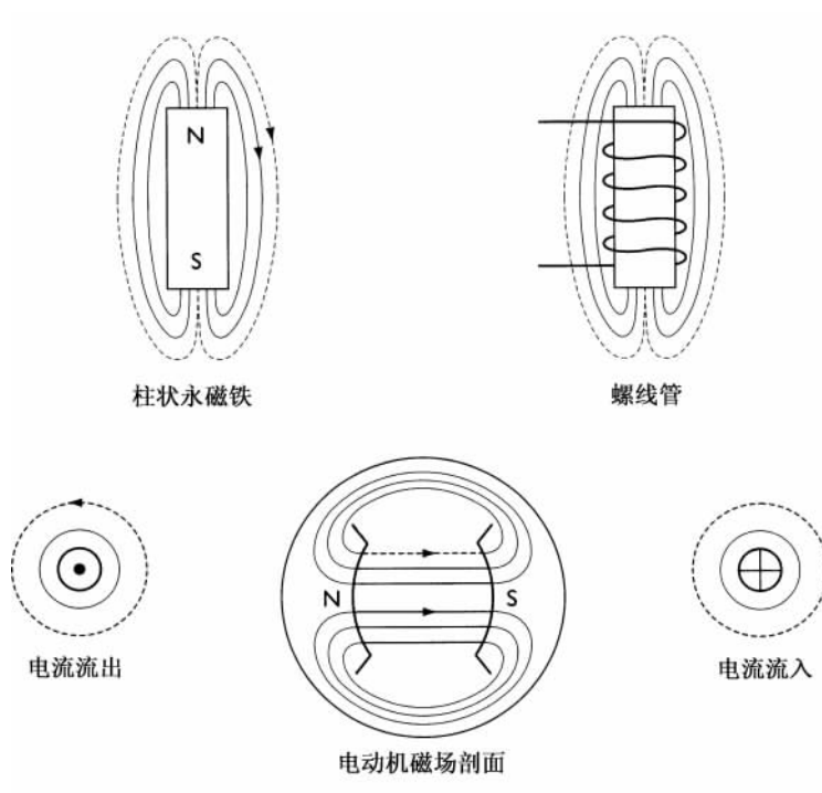
图 2.9 磁场
