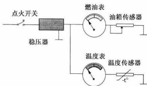
图 13.3 双金属片燃油表和温度表
