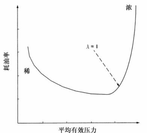
图 9.7 节气门位置不变时混合气浓度特性曲线
