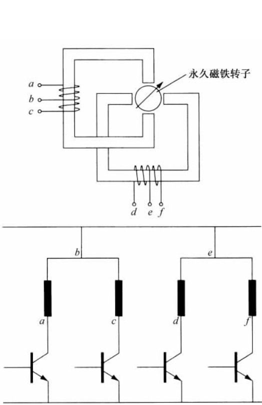
图 2.75 四相步进电机及其电路
