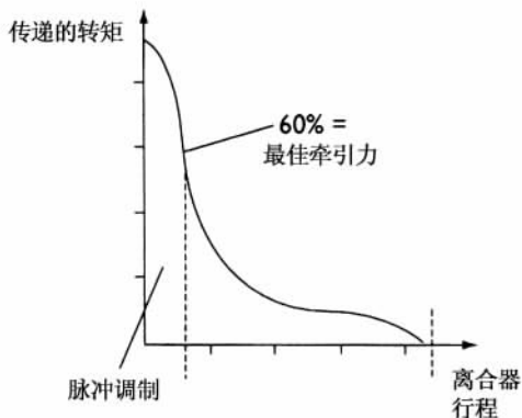
图 15.16 电控离合器系统传递转矩曲线图
