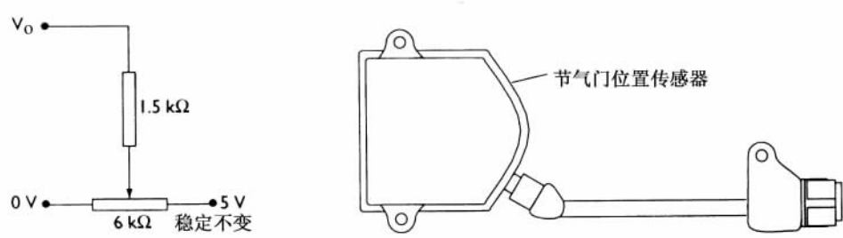
图 10.45 节气门位置传感器及其电路图
