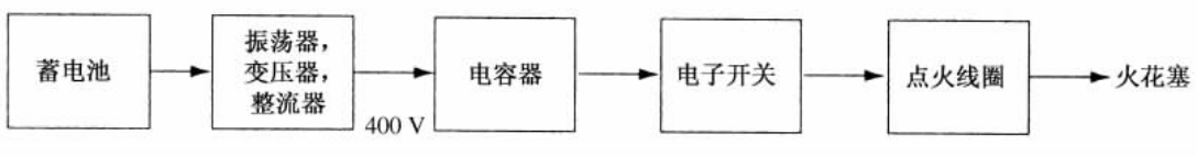
图 8.17 CDI 系统
