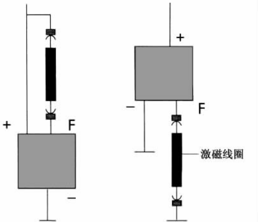
图 6.17 电压调节器的接线方式
