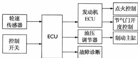
图 15.7 牵引控制系统方框图
