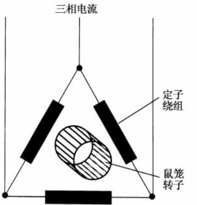
图 17.2 由许多磁极组成的鼠笼转子式异步电机
