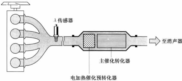
图 10.14 电加热催化预转化器
