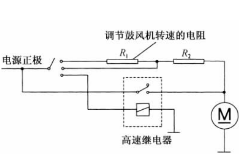
图 14.5 三速鼓风机控制系统电路图
