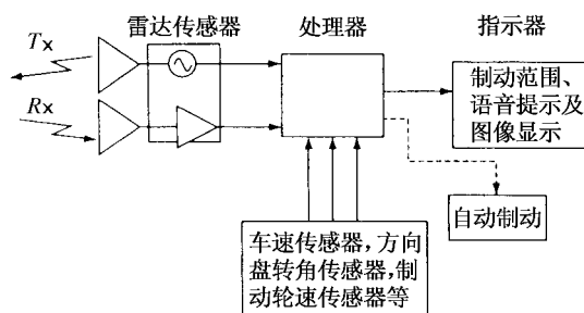
图 16.39 使用视觉增强系统的防碰雷达工作原理方框图
