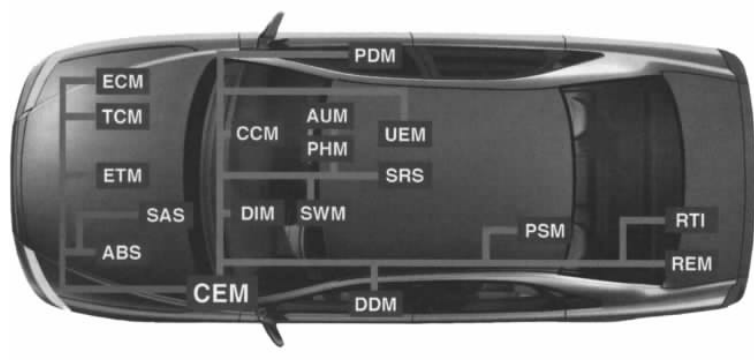
图 4.22 能够通讯的中央控制单元
