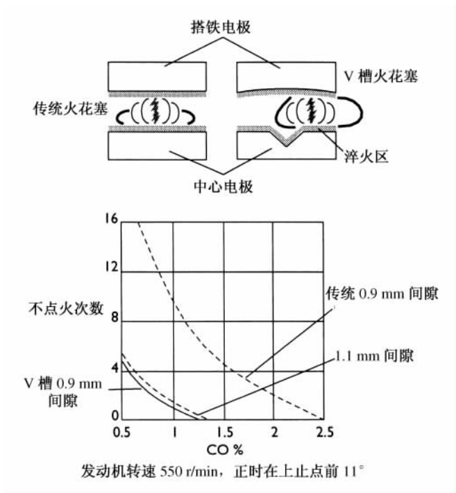
8.33 V 槽火花塞发火方式与传统火花塞相比的性能提高说明图
