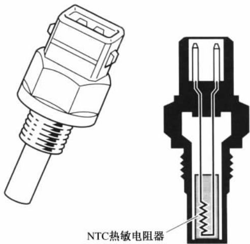
图 9.25 冷却液温度传感器
