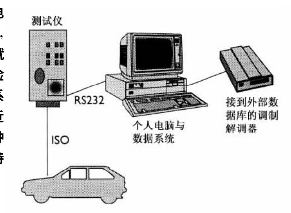
图 3.17 远程诊断
