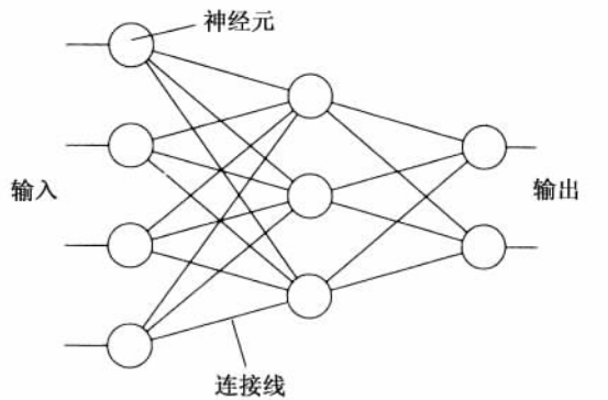
图 10.58 神经网络
