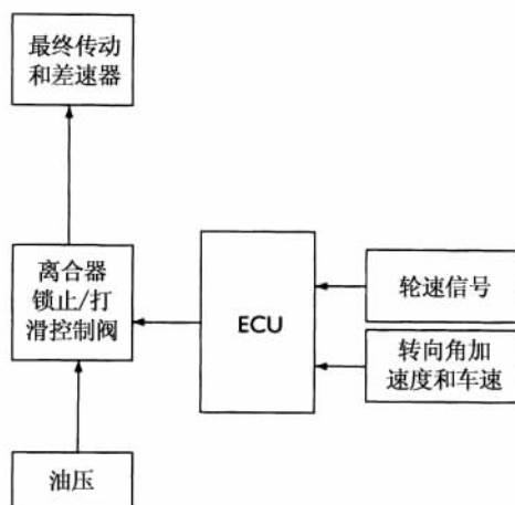
图 15.18 电控差速器控制方框图
