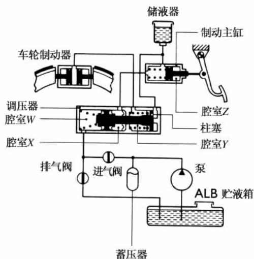
图 15.19 本田制动防抱死系统
