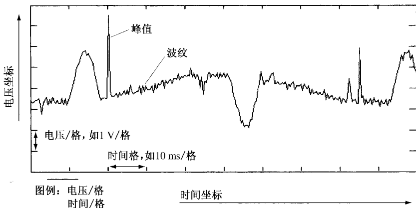
图 3.20 示波器识读
