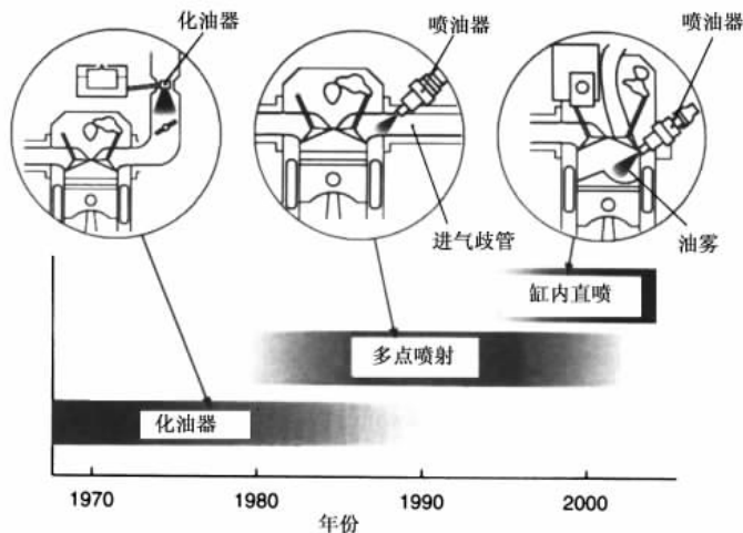
图 10.22 燃油供给系统的发展过程
