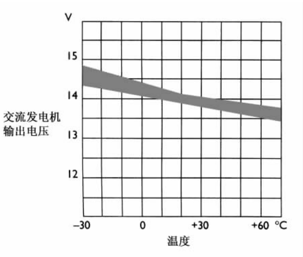
图 6.21 电压调节器的温度与电压之间的关系
