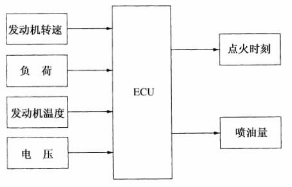
图 10.2 点火与燃油喷射控制系统
